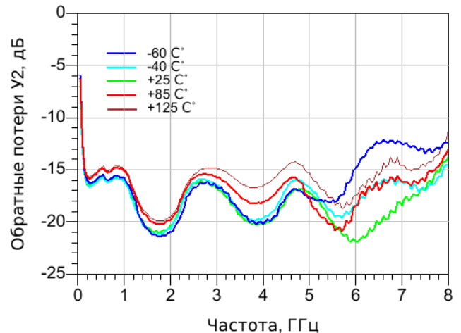
Обратные потери по выходу У2, дБ
