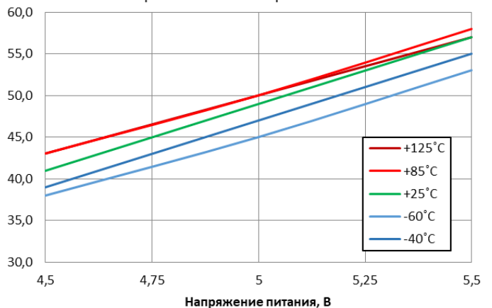
I_{\text{п}} , мА Ток потребления У1 от напряжения питания
