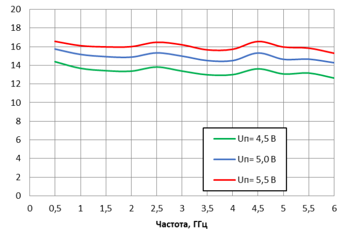
P_{\text{вых}} 1\text{дБ} , дБм Вых. точка компрессии 1дБ ШПУ1
