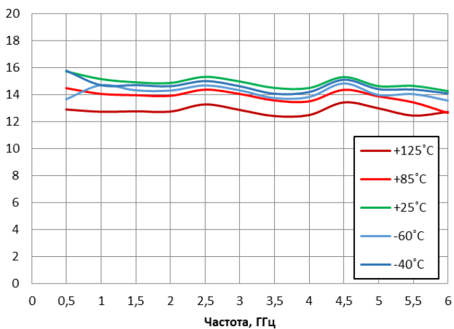
P_{\text{вых}} 1\text{дБ} , дБм Вых. точка компрессии ШПУ1
