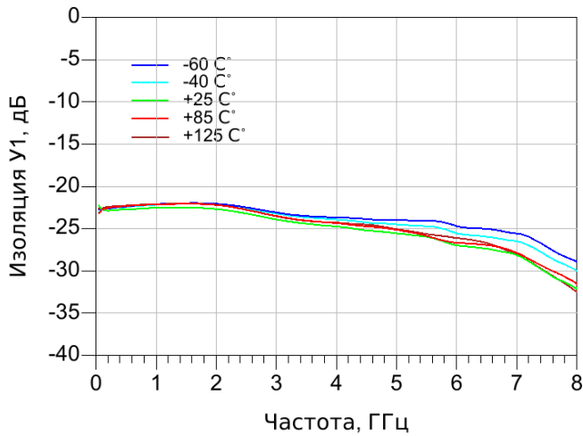
Изоляция У1, дБ
