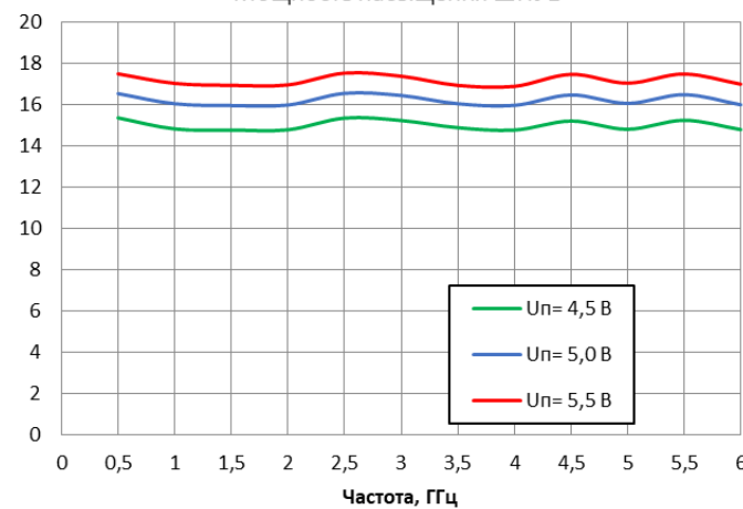
P_{\text{нас}} , дБм Мощность насыщения ШПУ1
