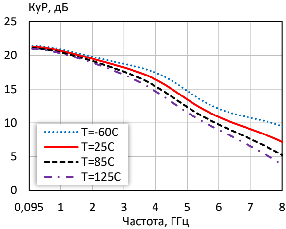
Коэффициент усиления при различной температуре ( I_p = 110 мА)
