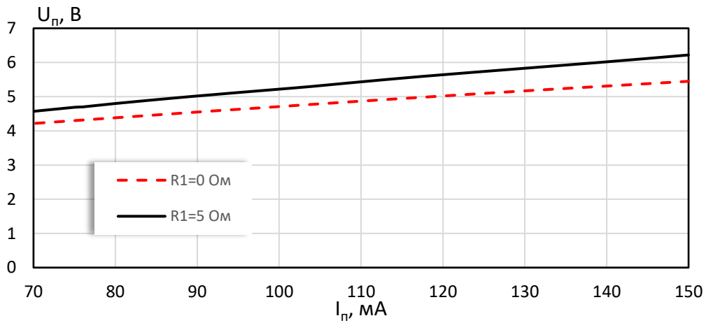
Зависимость напряжения питания от тока покоя для номиналов резистора R_1 = 0 \text{ Ом} и R_1 = 5 \text{ Ом}
