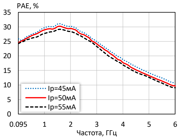
КПД по добавленной мощности в точке Р вых3дБ при различных режимных токах
