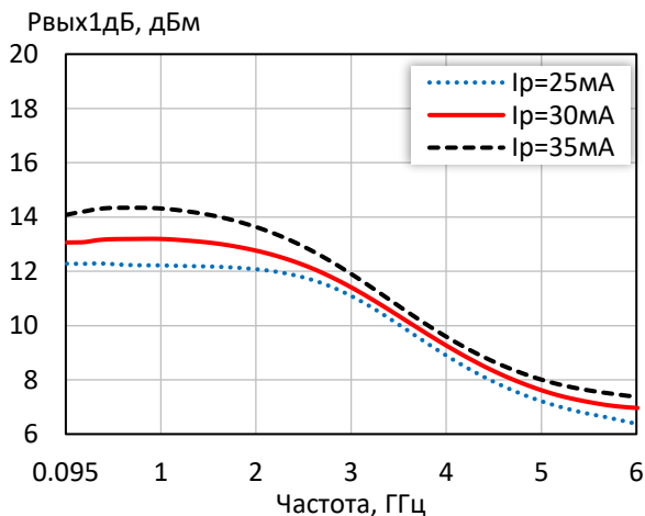
Выходная мощность при уровне компрессии K_{yP} на 1 дБ при различных режимных токах
