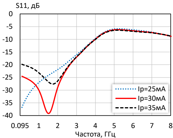
Коэффициент отражения от входа при различных режимных токах
