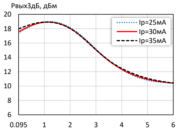
Выходная мощность при уровне компрессии K_{yP} на 3 дБ при различных режимных токах
