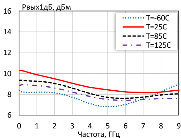
Выходная мощность при уровне компрессии K_{ур} на 1 дБ при различной температуре ( I_p = 30\text{ mA} )
