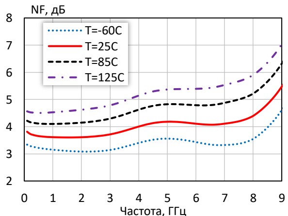
Коэффициент шума при различной температуре ( I_p = 30\text{ mA} )
