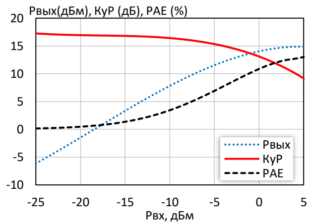
Выходная мощность, коэффициент усиления, КПД по добавленной мощности ( f = 3 ГГц, I_p = 30 мА)
