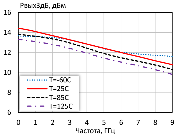
Выходная мощность при уровне компрессии K_{ур} на 3 дБ при различной температуре ( I_p = 30\text{ mA} )
