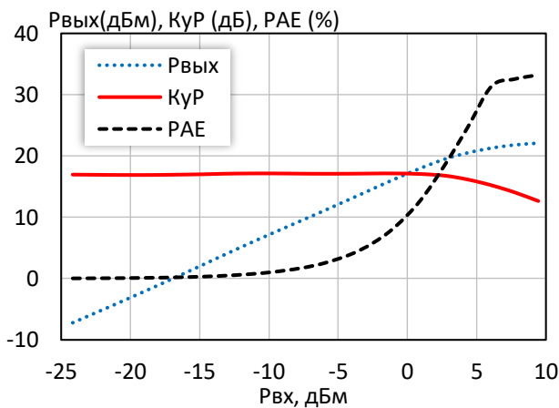
Выходная мощность, коэффициент усиления, КПД по добавленной мощности ( f = 10\text{ МГц} , I_p = 100\text{ мА} )
