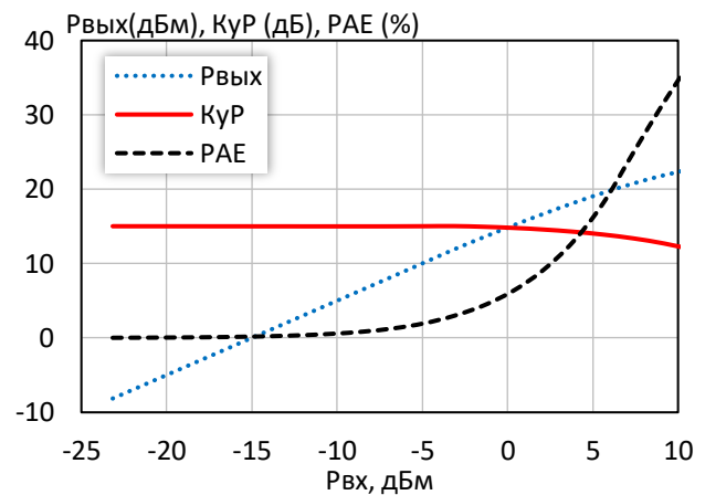
Выходная мощность, коэффициент усиления, КПД по добавленной мощности ( f = 3\text{ ГГц} , I_p = 100\text{ мА} )
