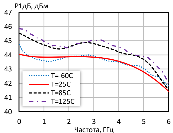
Выходная мощность при уровне компрессии K_{\text{уР}} на 1 дБ при различной температуре ( I_p = 130\text{ mA} )
