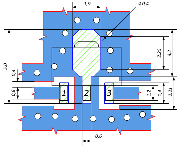
ПЛОЩАДКА ДЛЯ МОНТАЖА КОРПУСА КТ-47 (SOT-89)
