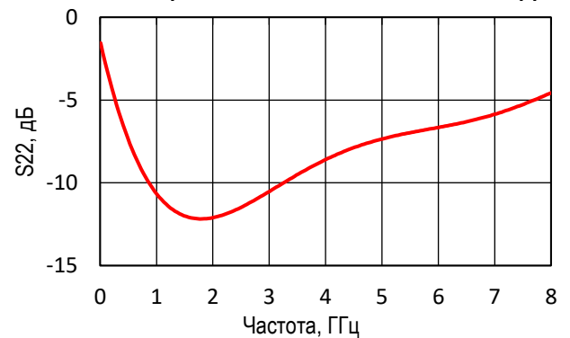
Рисунок 15 – Зависимость коэффициента отражения по выходу «TERM» от частоты
