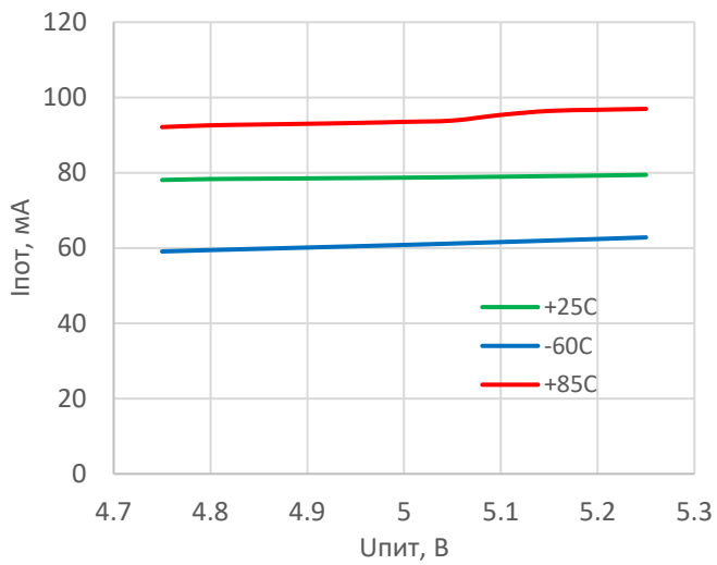
Ток потребления
