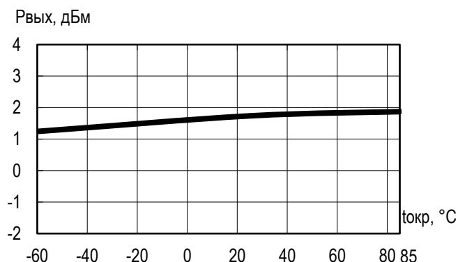
Зависимость мощности выходного сигнала от температуры ( U_n = 5\text{ В} , P_{вх} = 0\text{ дБм} )
