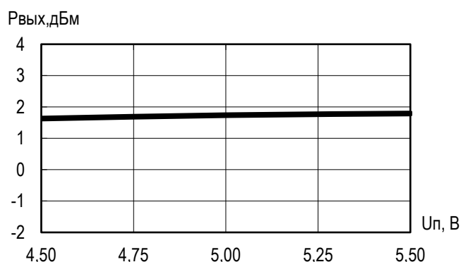
Зависимость мощности выходного сигнала от напряжения питания ( U_n = 5\text{ В} , P_{вх} = 0\text{ дБм} )
