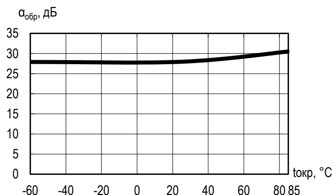
Зависимость обратной изоляции от температуры ( U_n = 5\text{ В} , P_{вх} = 0\text{ дБм} )
