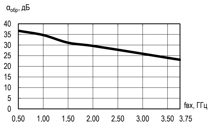
Зависимость обратной изоляции от частоты входного сигнала ( U_n = 5\text{ В} , P_{вх} = 0\text{ дБм} )
