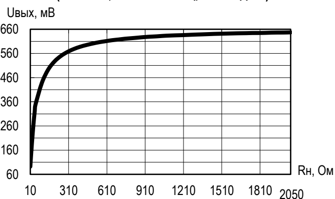
Зависимость амплитуды основной гармоники в спектре выходного сигнала от сопротивления нагрузки ( U_n = 5\text{ В} , f_{вх} = 500\text{ МГц} , P_{вх} = 0\text{ дБм} )
