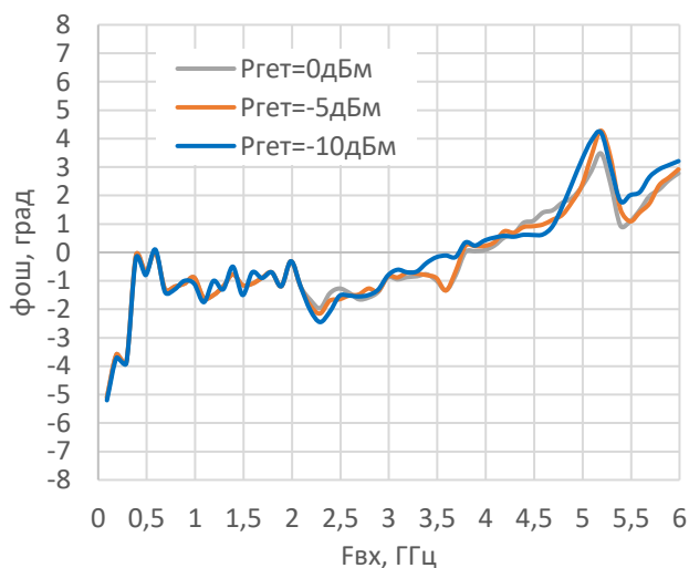
Фазовая ошибка фоз ( F_{\text{вх}} , P_{\text{гет}} )
