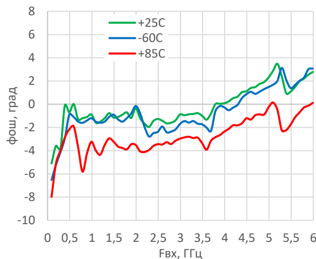
Фазовая ошибка фоз ( F_{\text{вх}} , T_{\text{окр}} )
