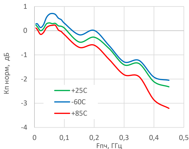
Нормированный коэффициент передачи K_{п\text{ норм}}(F_{пч}, T_{окр})
