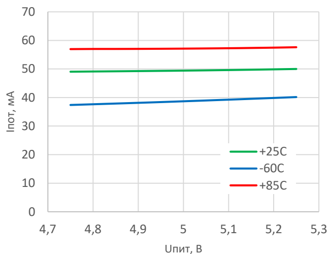
Ток потребления
