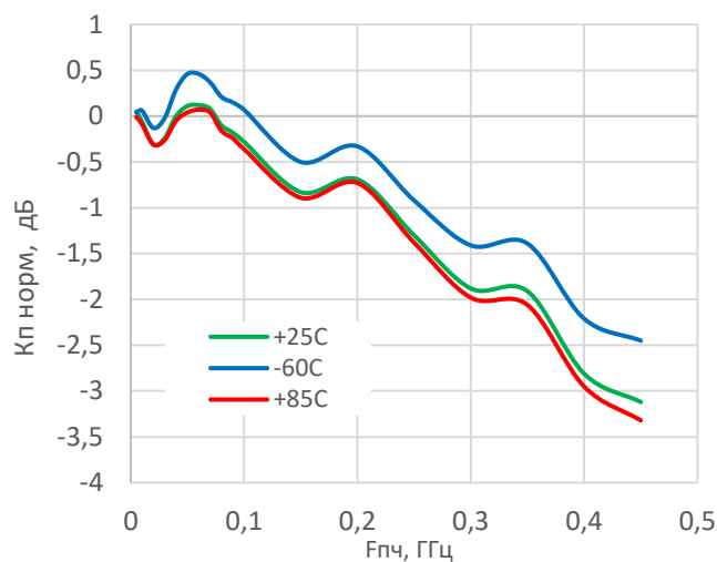
Нормированный коэффициент передачи Кп норм ( F_{пч} , T_{окр} )
