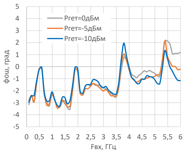
Фазовая ошибка фох ( F_{вх} , P_{гет} )
