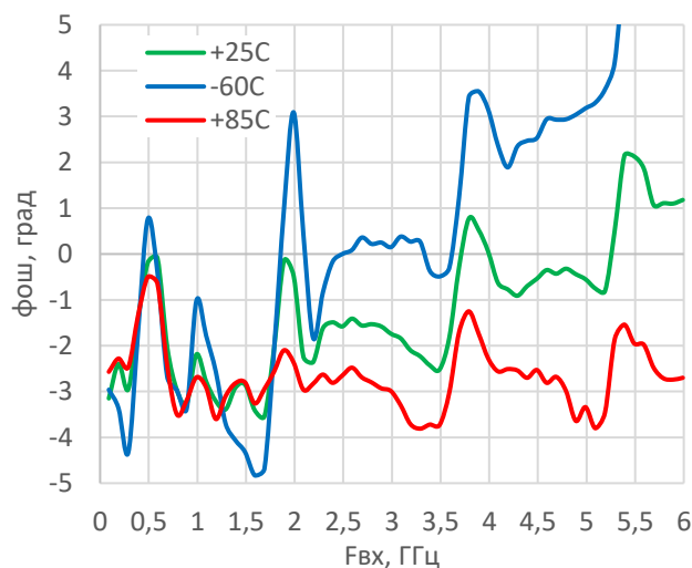
Фазовая ошибка фох ( F_{вх} , T_{окр} )
