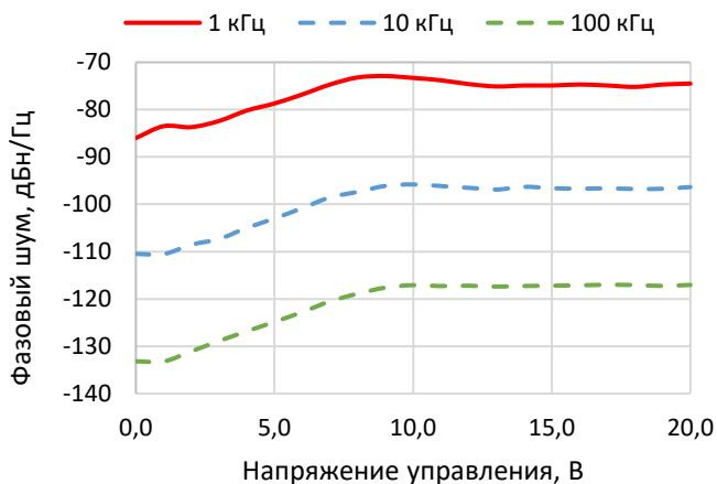
Рисунок 5 – фазовый шум
