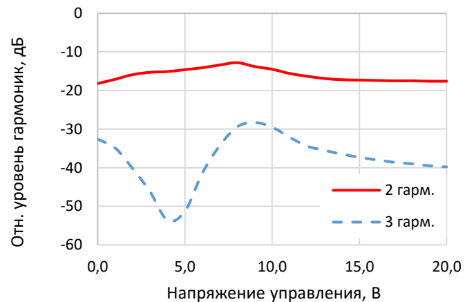
Рисунок 4 – относительный уровень гармоник
