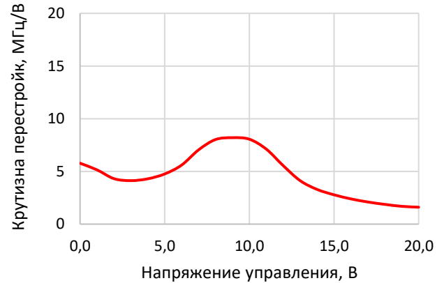
Рисунок 2 – крутизна перестройки
