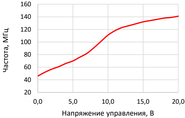
Рисунок 1 – диапазон перестройки
