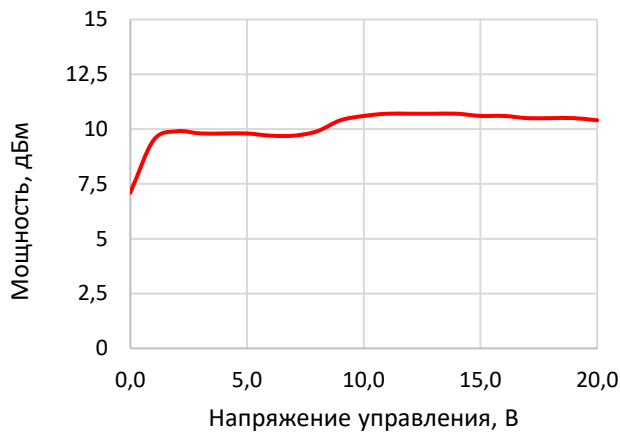
Рисунок 3 – выходная мощность
