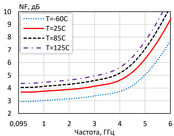
Коэффициент шума при различной температуре ( I_p = 110\text{ mA} )
