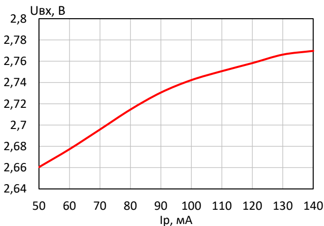
Входное напряжение покоя U_{\text{вх}} при изменении режимного тока I_p
