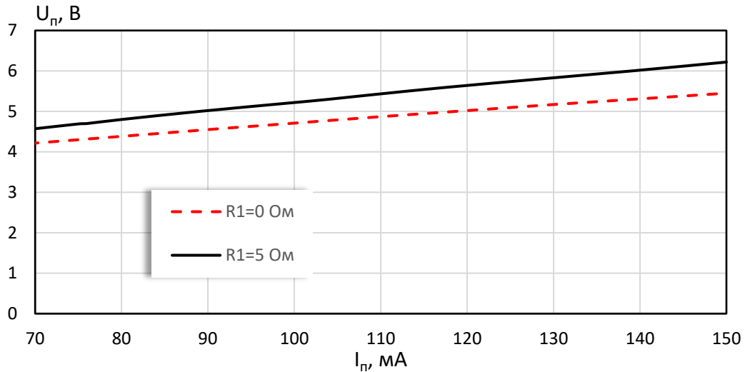
Зависимость напряжения питания от тока покоя для номиналов резистора R_1 = 0 \text{ Ом} и R_1 = 5 \text{ Ом}
