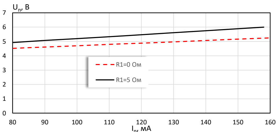
Зависимость напряжения питания от тока покоя для номиналов резистора R_1 = 15 \text{ Ом} и R_1 = 0 \text{ Ом}
