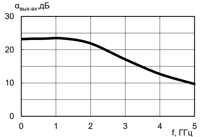
Зависимость изоляции выход-вход от частоты ( U_n = 5 В; I_p = 100 мА)
