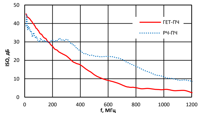
Зависимость изоляции РЧ-ПЧ от частоты РЧ ( I_p = 110 мА, P_{рч} = -20 дБм, P_{гет} = 0 дБм, f_{пч} = 100 МГц)
