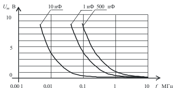
Рис. 6. Зависимости максимальной амплитуды выходного напряжения от частоты сигнала и ёмкости интегратора
