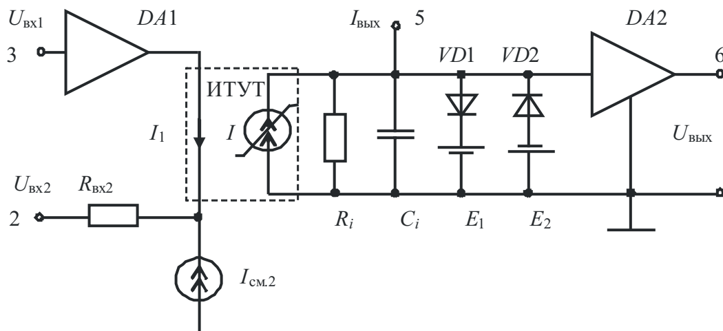
Рис. 1. Нелинейная эквивалентная схема CFOA типа AD844
