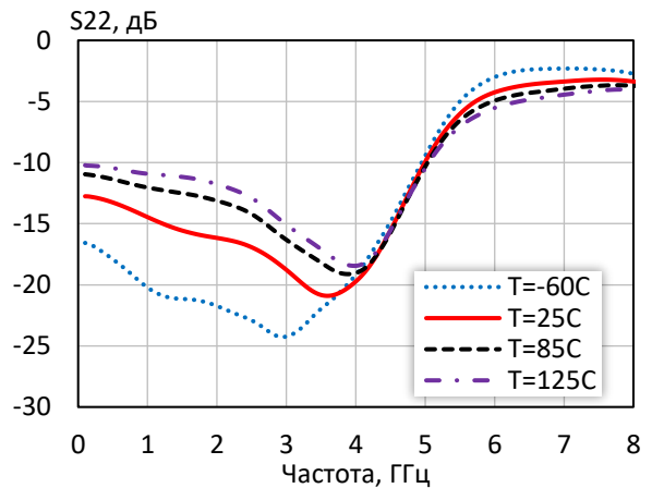
Кoeffициент отражения от выхода при различной температуре ( I_p = 30 мА)
