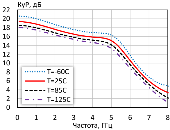
Кoeffициент усиления при различной температуре ( I_p = 30 мА)
