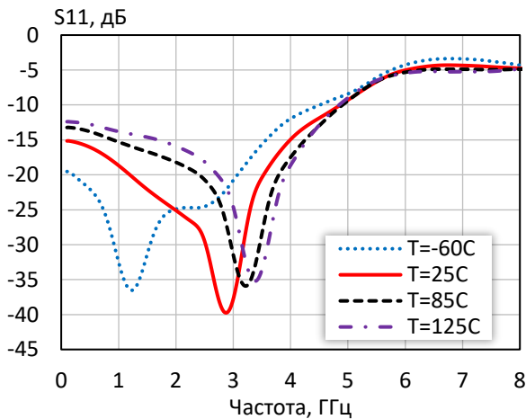
Кoeffициент отражения от входа при различной температуре ( I_p = 30 мА)
