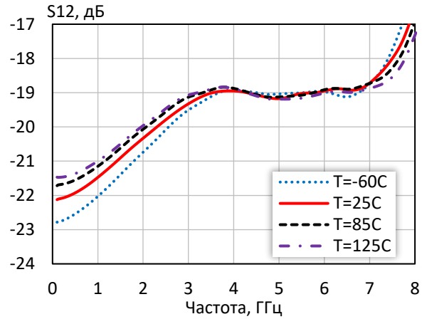
Кoeffициент обратной передачи при различной температуре ( I_p = 30 мА)
