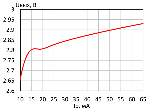
Выходное напряжение покоя U_{вых} при изменении режимного тока I_p
