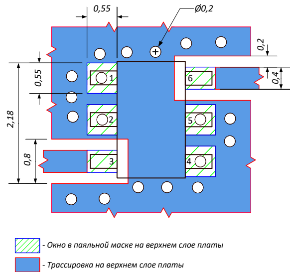
ПЛОЩАДКА ДЛЯ МОНТАЖА КОРПУСА 4337.6-1
