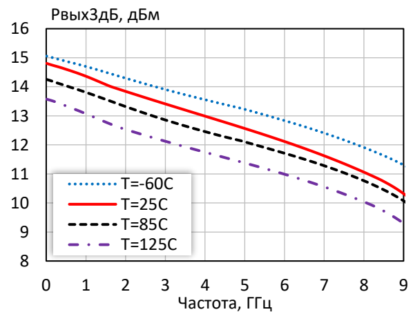
Выходная мощность при уровне компрессии K_{ур} на 3 дБ при различной температуре ( I_p = 30\text{ mA} )
