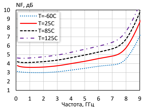
Коэффициент шума при различной температуре ( I_p = 50\text{ mA} )
