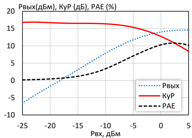
Выходная мощность, коэффициент усиления, КПД по добавленной мощности ( f = 3\text{ ГГц} , I_p = 30\text{ мА} )
