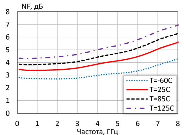
Коэффициент шума при различной температуре ( I_p = 100\text{mA} )
