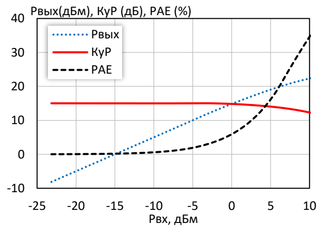
Выходная мощность, коэффициент усиления, КПД по добавленной мощности ( f = 3\text{ ГГц} , I_p = 100\text{ mA} )
