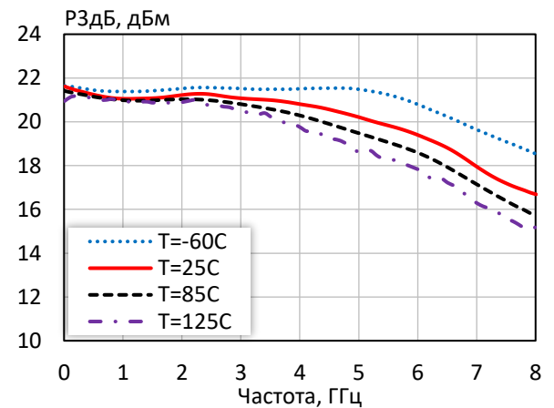
Выходная мощность при уровне компрессии K_{ур} на 3 дБ при различной температуре ( I_p = 100\text{mA} )
