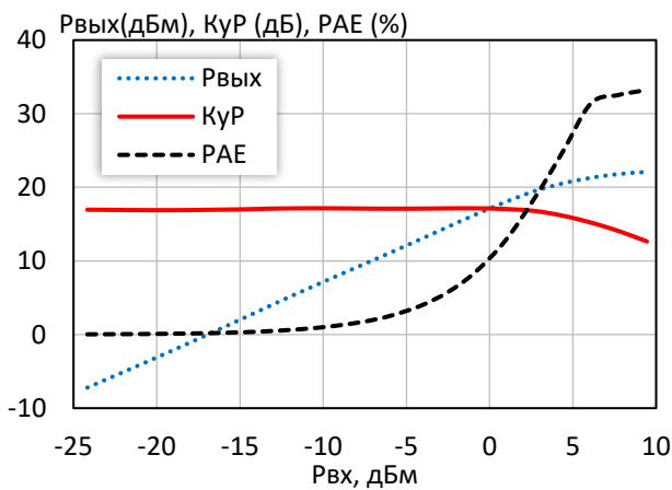
Выходная мощность, коэффициент усиления, КПД по добавленной мощности ( f = 10\text{ МГц} , I_p = 100\text{ mA} )
