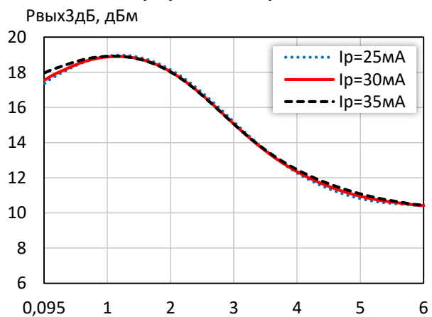
Выходная мощность при уровне компрессии K_{up} на 3 дБ при различных режимных токах
