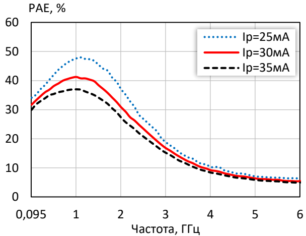
КПД по добавленной мощности в точке P_{\text{вых3дБ}} при различных режимных токах
