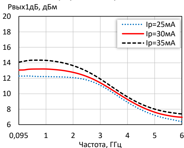
Выходная мощность при уровне компрессии K_{up} на 1 дБ при различных режимных токах
