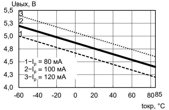
Зависимость напряжения на выходе от температуры ( I_p = 80\text{ mA}; 100\text{ mA}; 120\text{ mA} )
