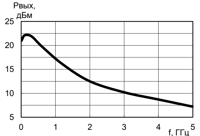
Зависимость выходной мощности от частоты ( U_n = 5 В; I_p = 100 мА; P_{вх} = 6 дБМ)
